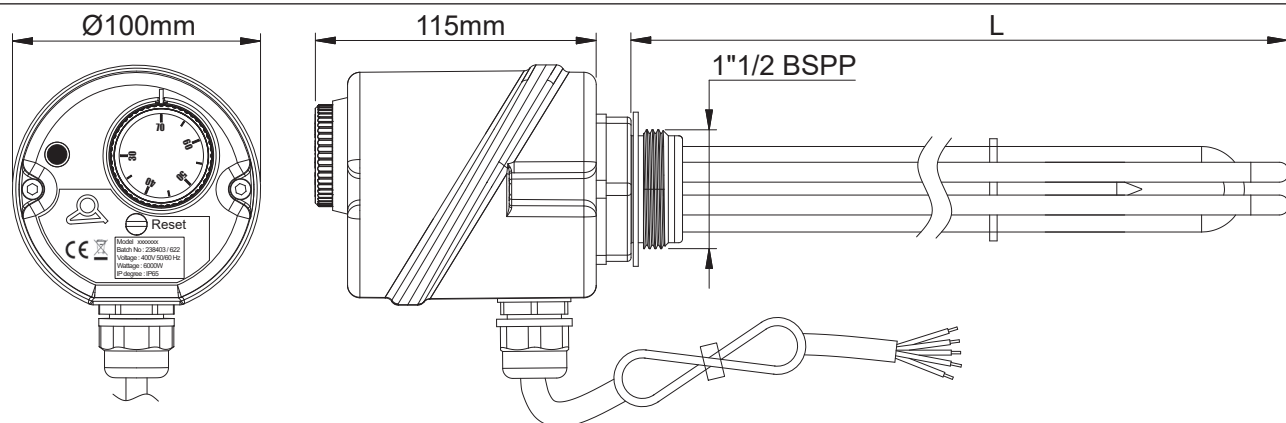
3-poliger 400V-Heizer
